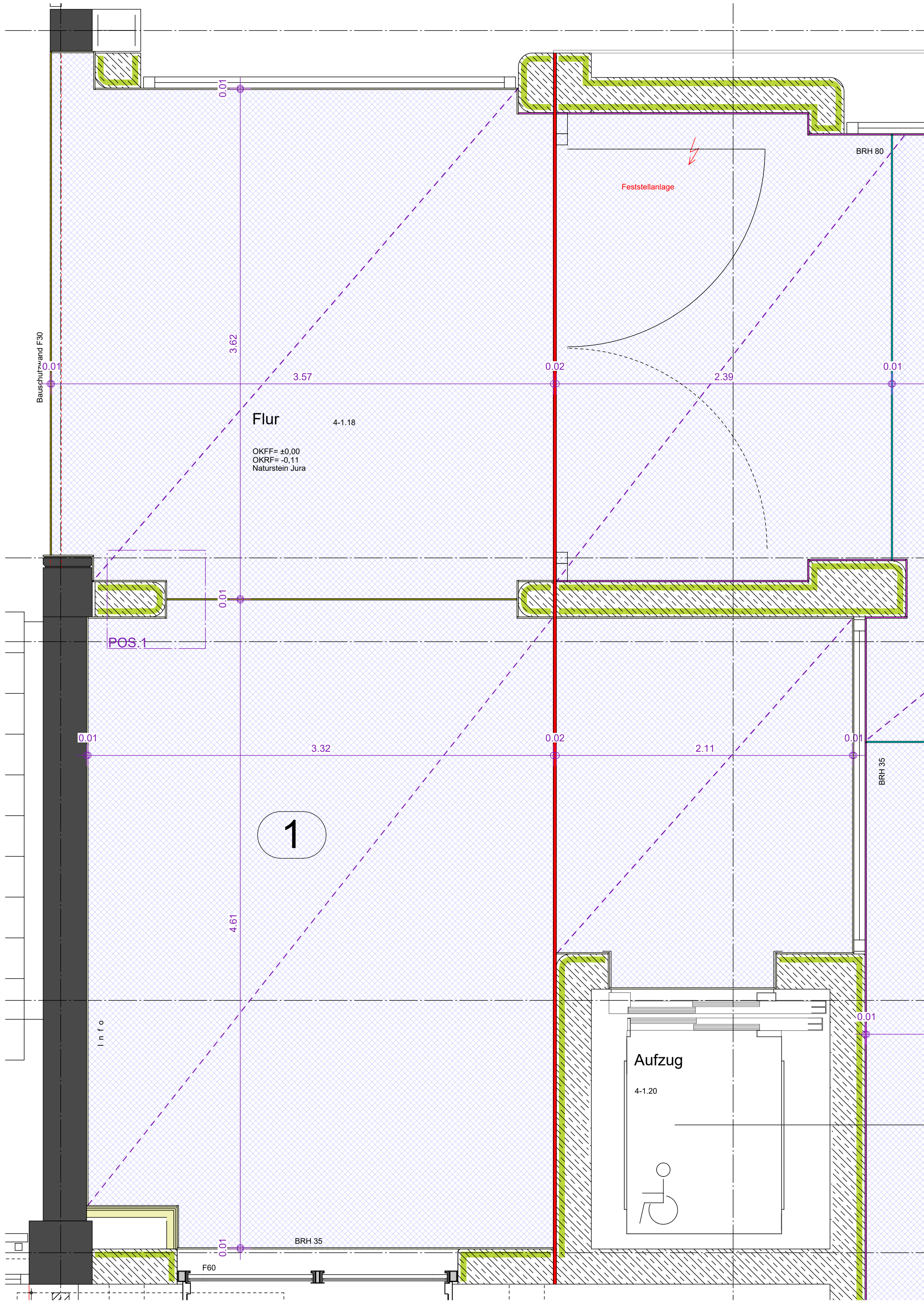
EG GRUNDRISSAUSSCHNITT ESTRICHARBEITEN FLUR 4-1.18 M 1:20
